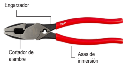
Engarzador
